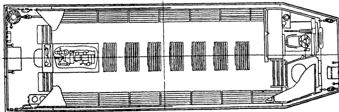
Главная палуба
