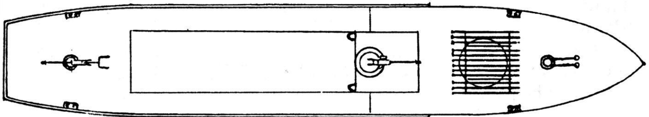
План палубы
