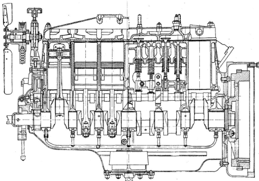
Продольный разрез двигателя ЗИС-5
