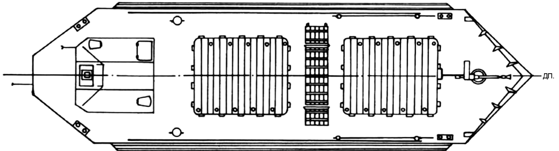
Плaшкoут двyхтрyмный
