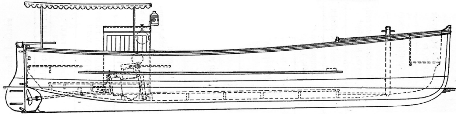
Разрез по моторному отсеку
