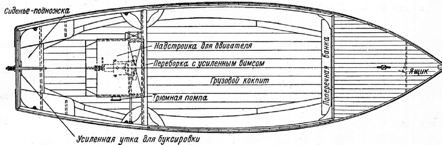
План трюма
