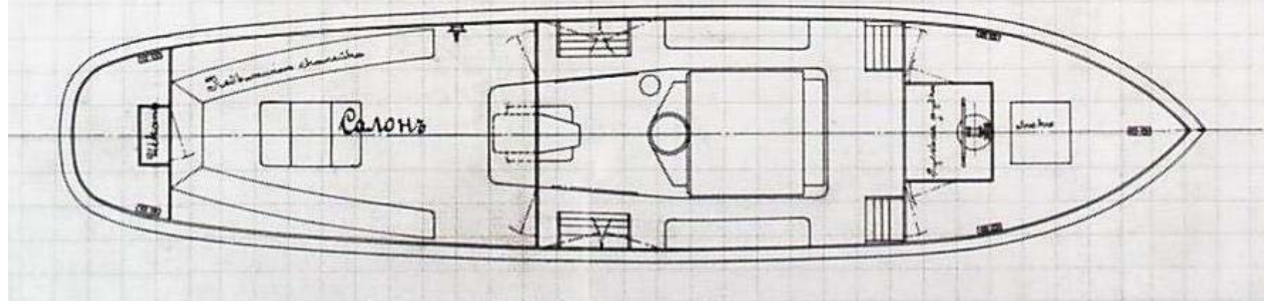
План на уровне главной палубы
