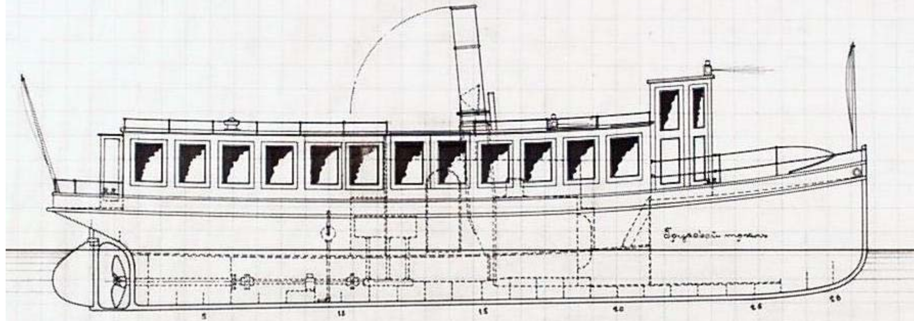
Вид на правый борт
