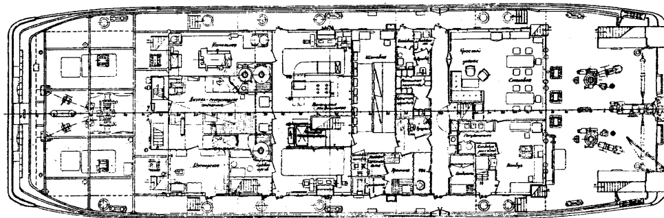
Главная палуба
